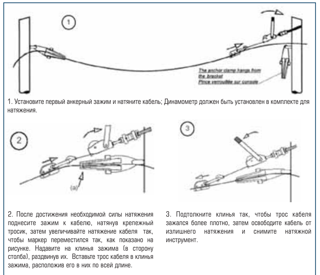
Рис. 2. Способ монтажа кабеля с помощью зажима «МАЛИКРО»
