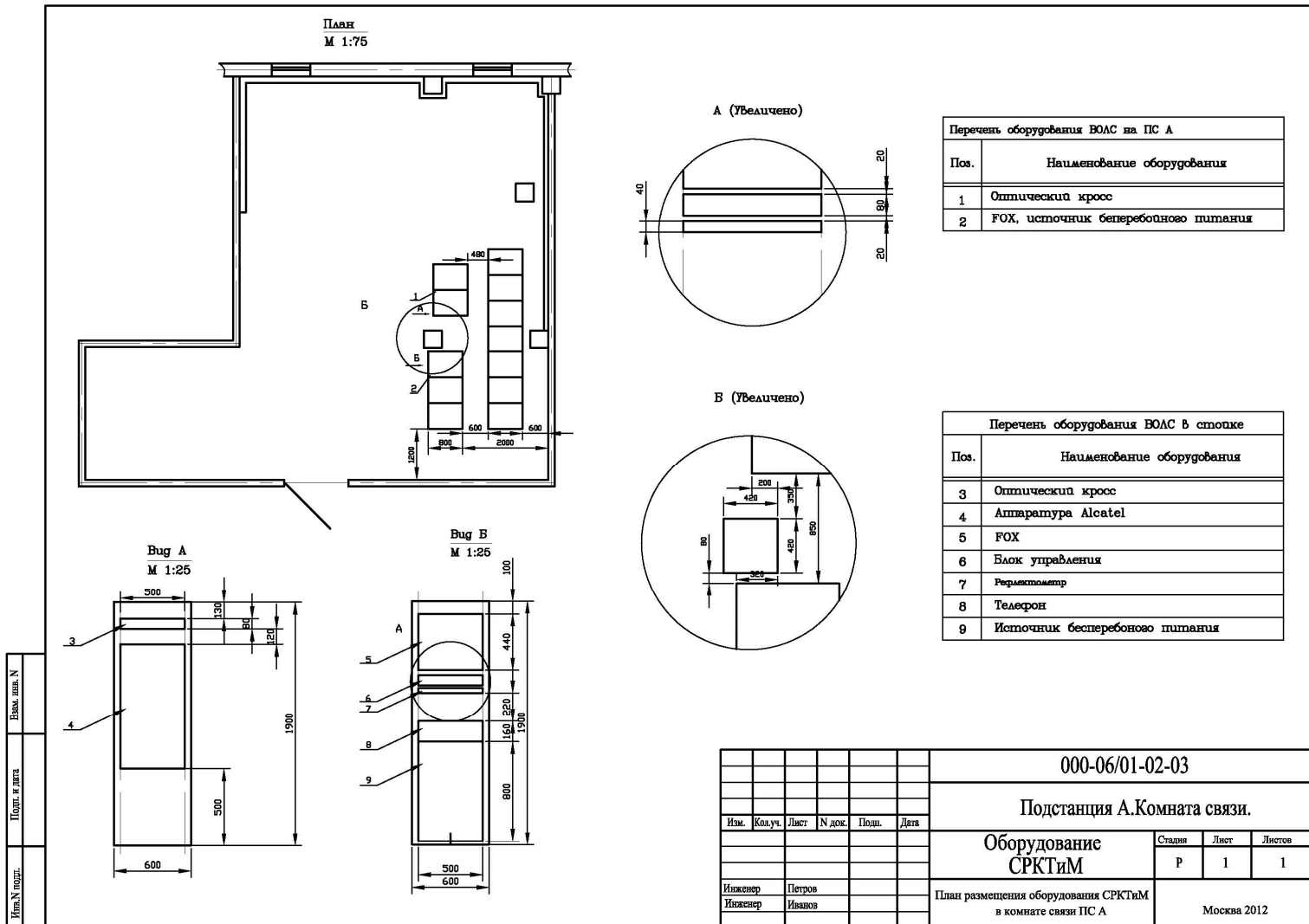
Рисунок А.28 Схема расположения оборудования СРКТиМ на ПС А
