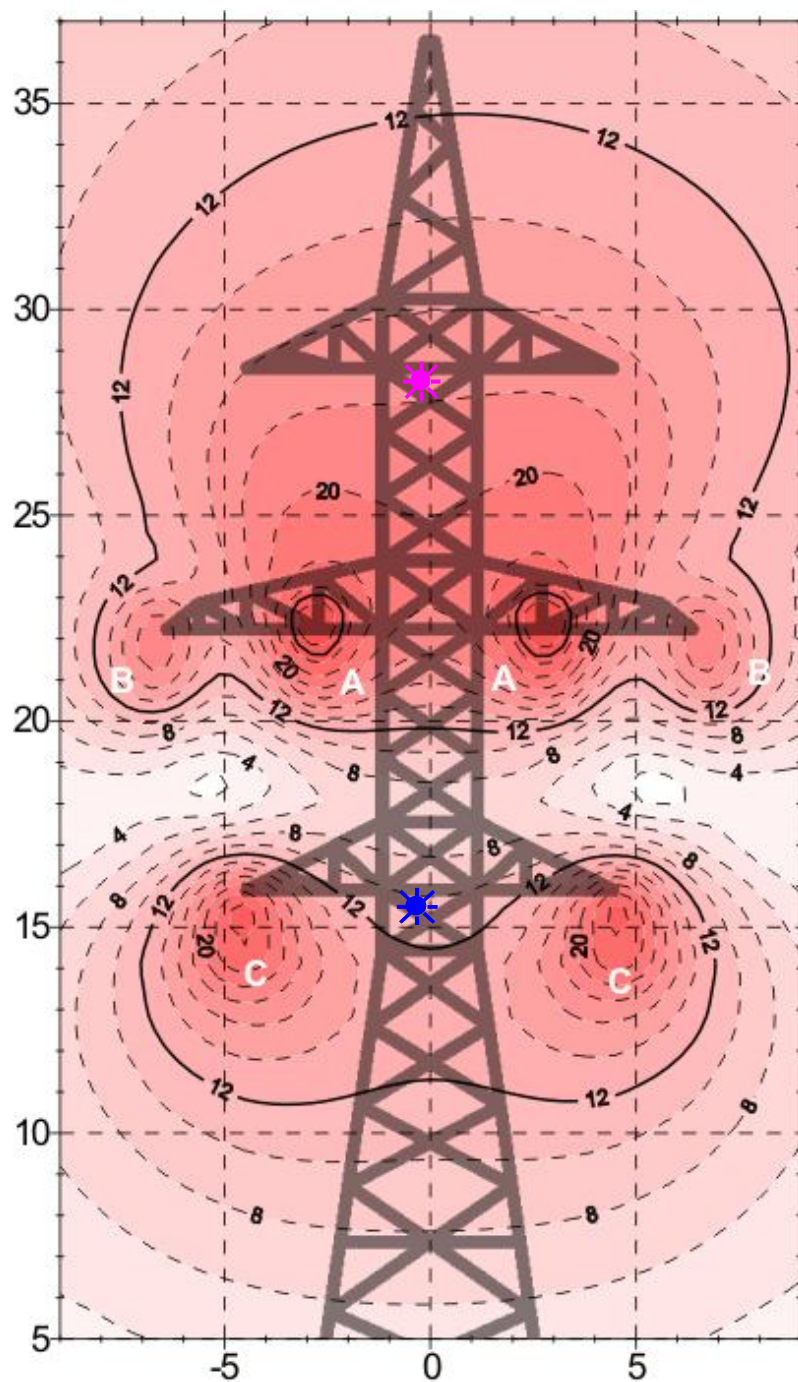
Рисунок А.16 Расчет наведенного потенциала электрического поля в плоскости А
