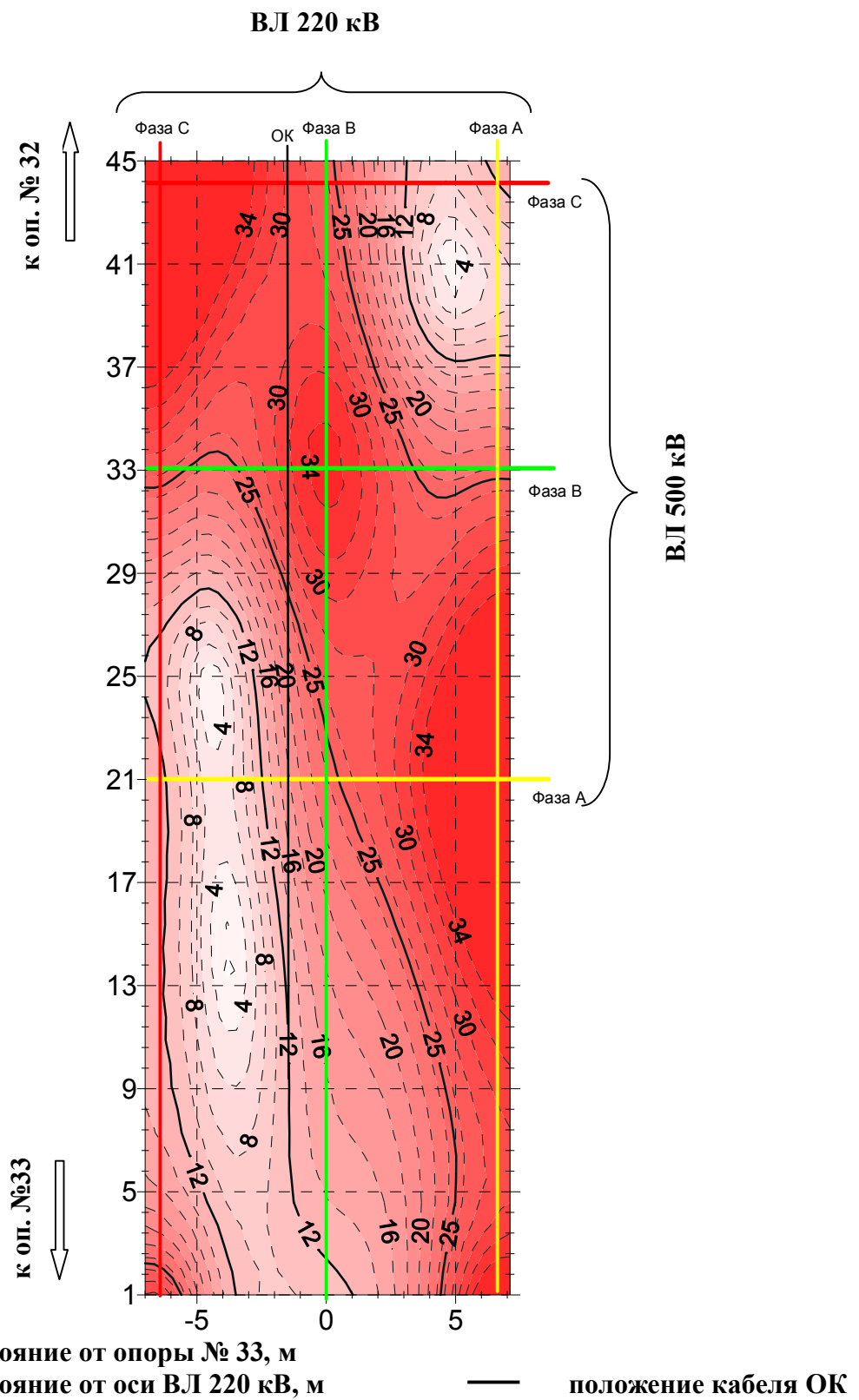
Рисунок А.21 Наведенный потенциал электрического поля в плоскости В в месте пересечения ВЛ 220 кВ с ВЛ 500 кВ
