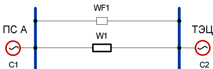
Рисунок А.1 - Расчетная схема для ВЛ 110 кВ ПС А – ТЭЦ
